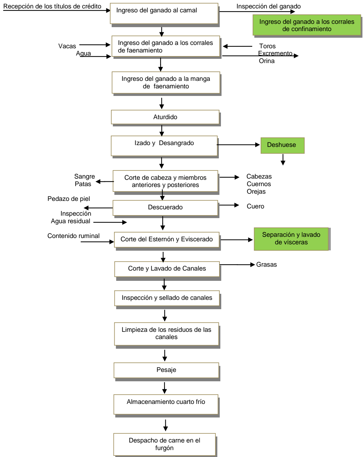
Gráfico 1. Procesos de faenamiento en el camal municipal de Otavalo Fuente: Administración Camal Municipal de Otavalo (2012)
