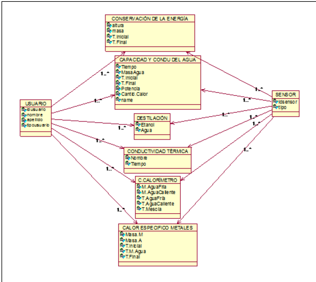
Figura 27 Diagrama de clases con atributos aplicado al Sistema de entrenamiento y enseñanza experimental
