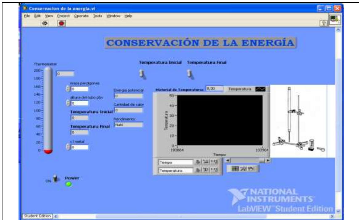
Figura 29 Conservación de la energía
