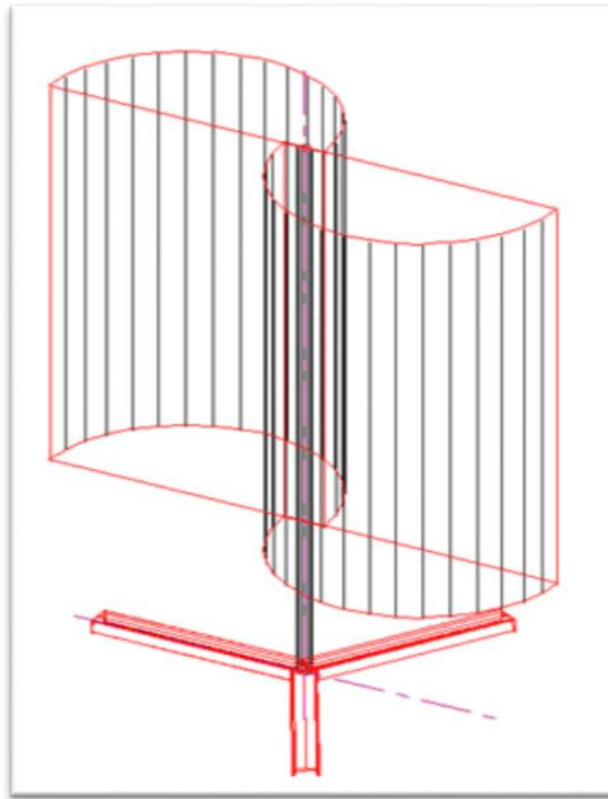
Figura 6: Rotor y el eje.
