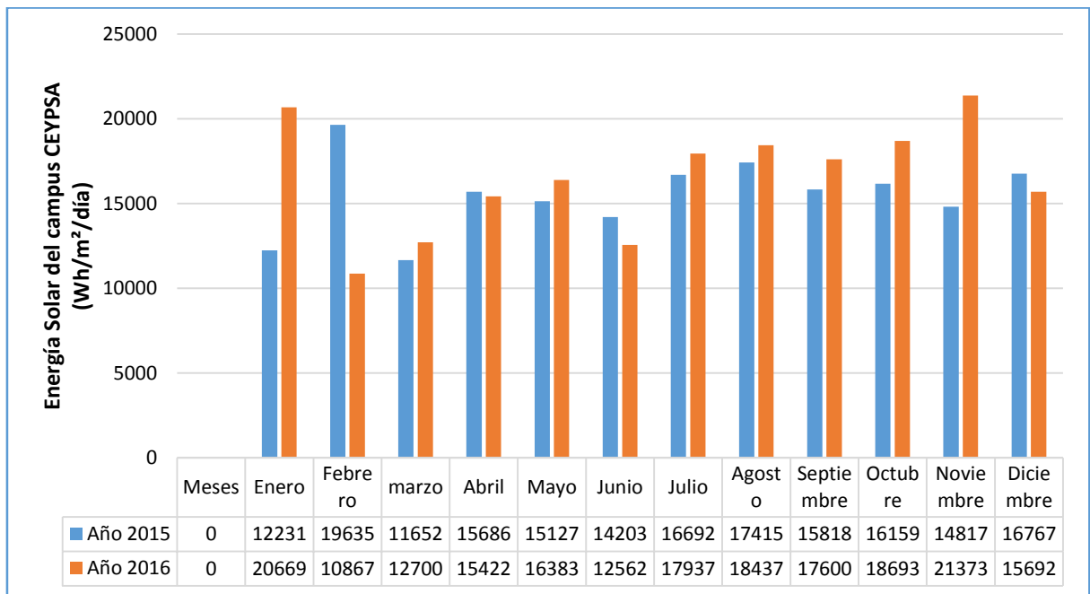
Figura 17: Potencial Energético Solar del campus CEYPSA.
