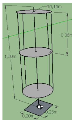
Figura 22: Aerogenerador de eje vertical tipo savonius.
