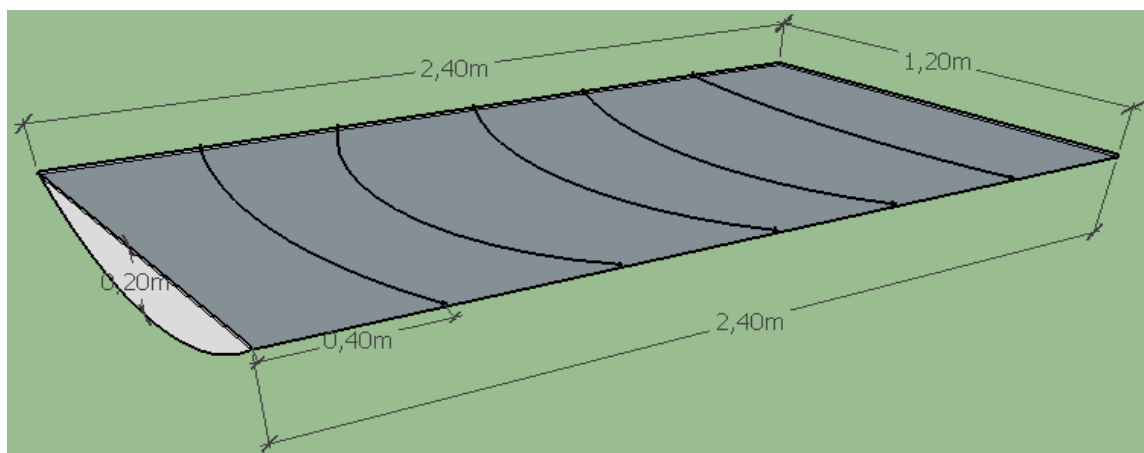
Figura 20: Soporte de la lámina de acero inoxidable.
