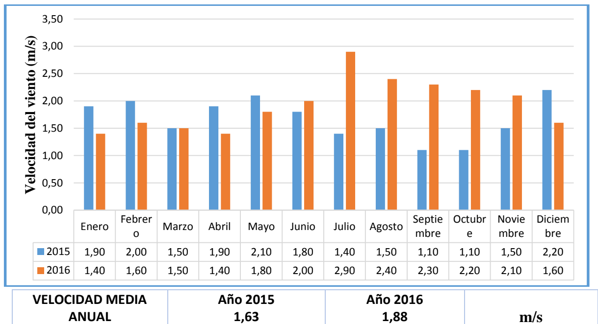
Figura 18: Velocidad media anual del viento en el campus CEYPSA.
