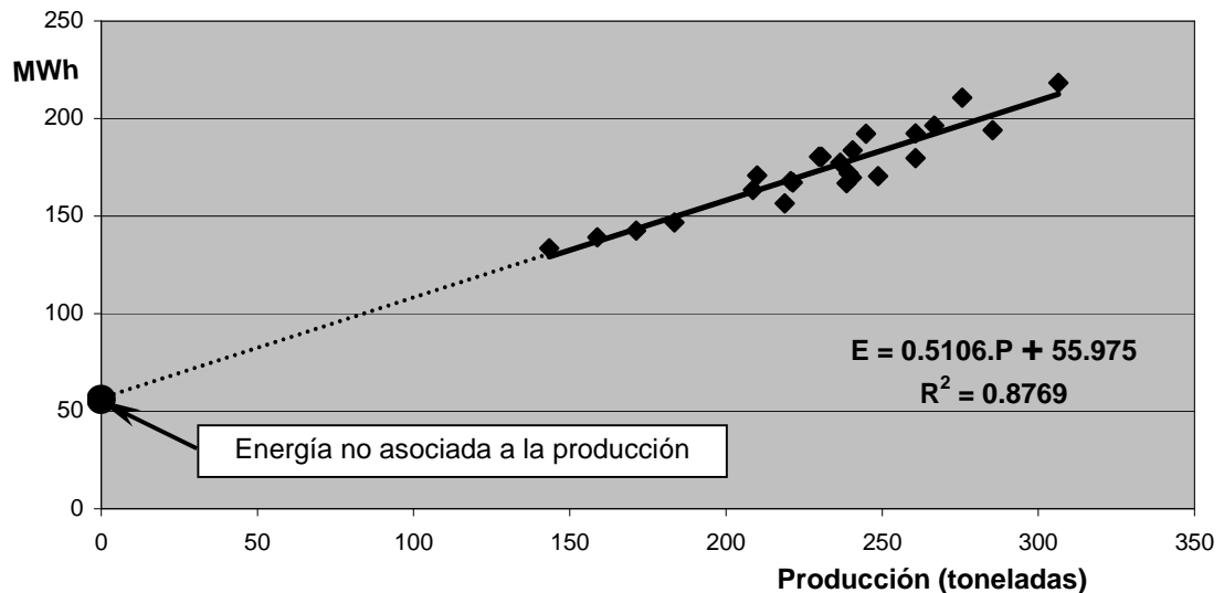
Diagrama de Consumo Electricidad vs. Producción
