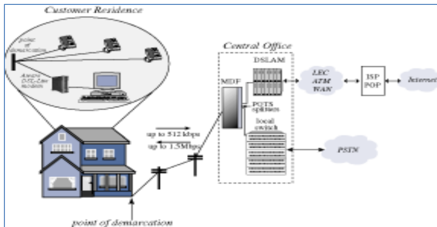
Figura 1.9: ADSL residencial.
