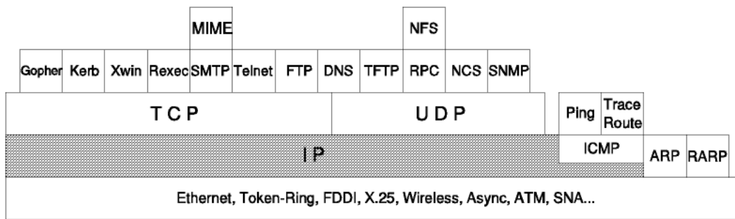
Gráfico 3: Estructura de un datagrama IP
