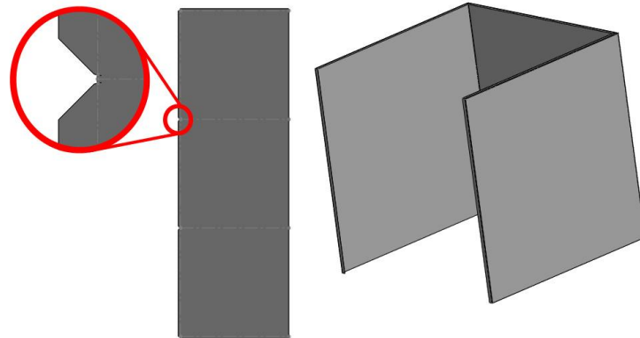
Fig. 3.13. Representación del modelo 3D de la chapa de acero inoxidable utilizada en el ensamblaje del prototipo de horno.
