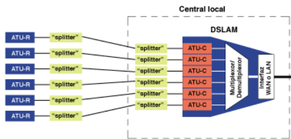
Figura 1.7: Estructura de un armario DSLAM.
