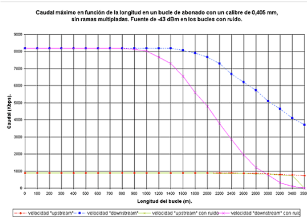
Figura 1.6: Relación Caudal máximo- Distancia a la central.
