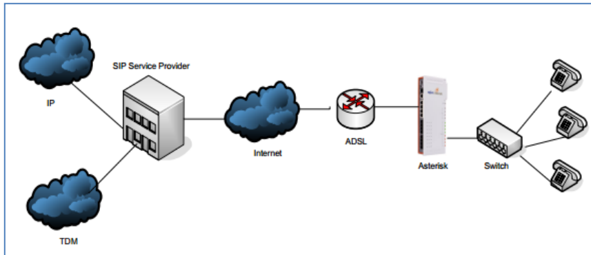
Figura 3.4.: Diseño de la red con VoIP
