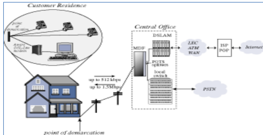
Figura 1.9: ADSL residencial.
