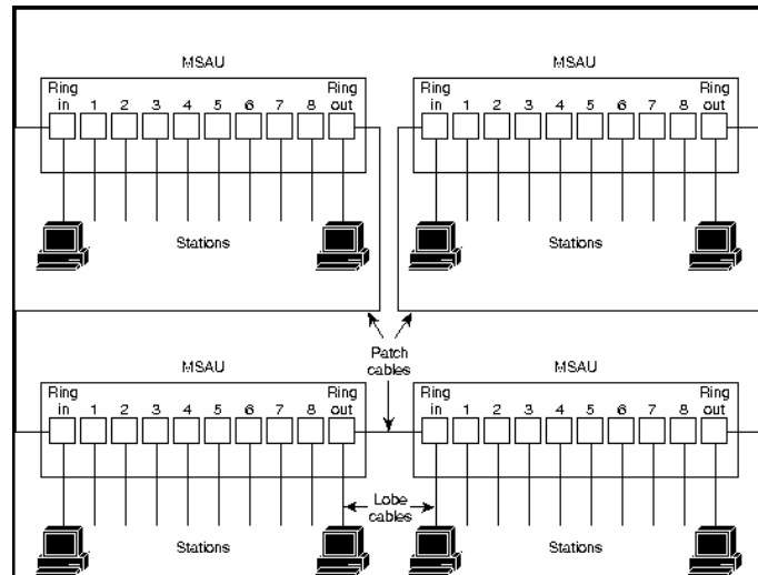
Figura 1.1: Conexiones Físicas
