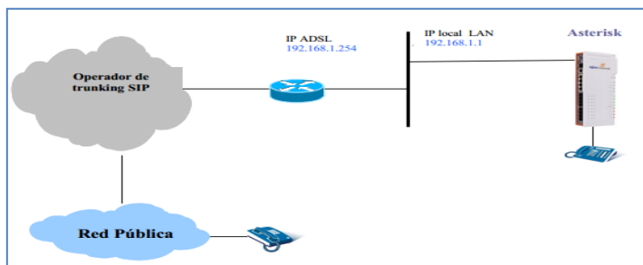
Figura 3.5.: Diseño de la red con VoIP
