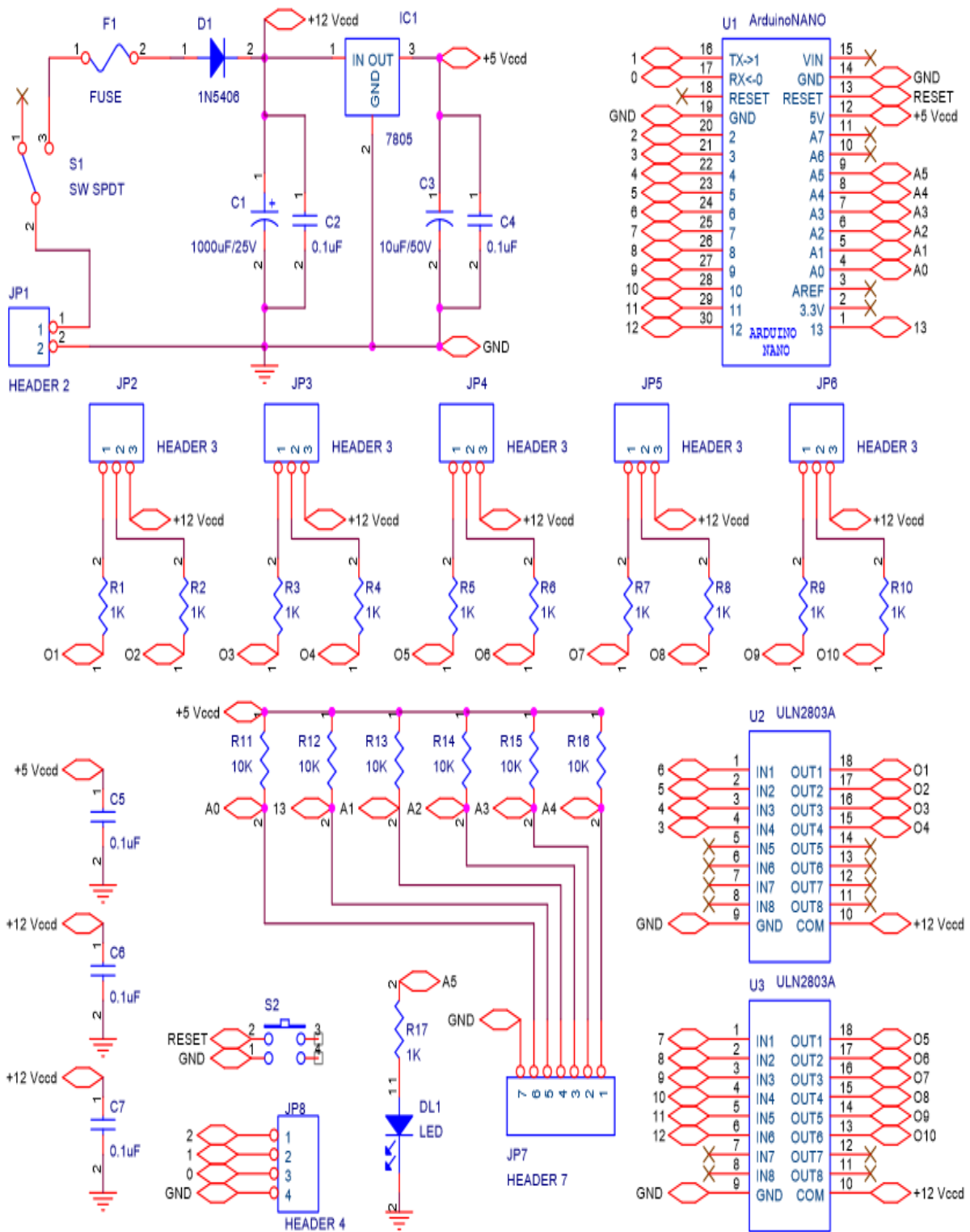
Figura 16: Diagrama electrónico
