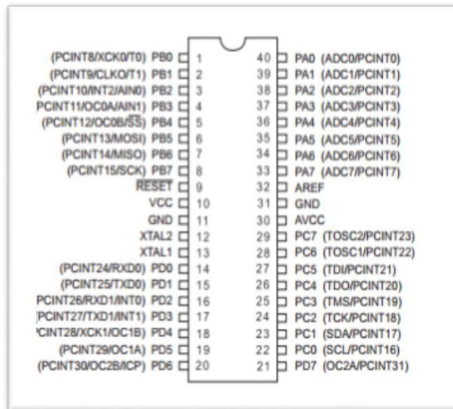
Figura 26: ATmega164A
