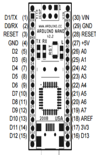
Figura 23: Datasheet de Arduino nano
