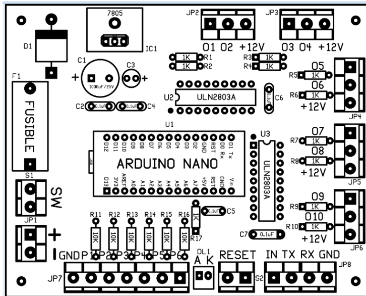
Figura 21: Elementos Electrónicos primer nivel
