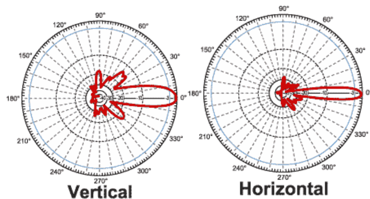
PATRONES DE GANANCIA RF DE LA ANTENA
