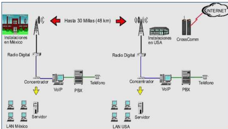
FIGURA 1.17 ENLACE DE EQUIPOS INALÁMBRICOS
