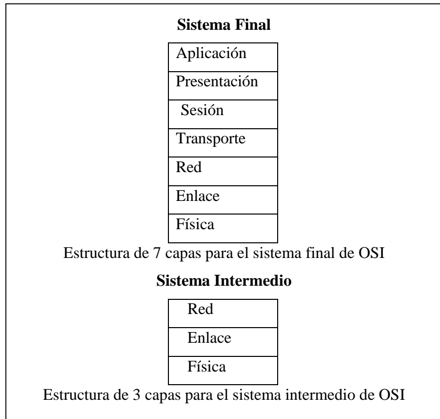
FIGURA 1.9 MODELO OSI
