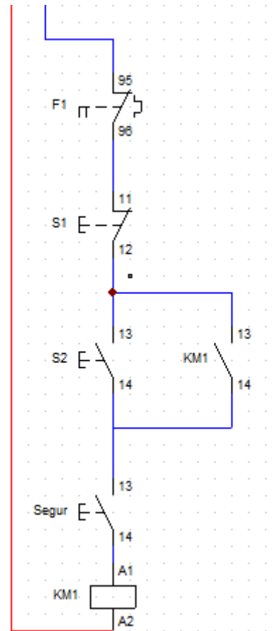
ANEXO H CIRCUITO DE CONTROL
