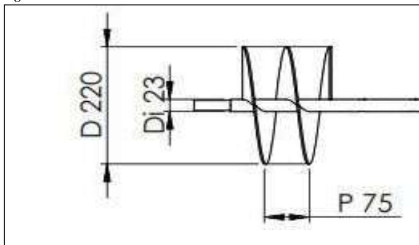
Figura N° 18: Nomenclatura de tornillo sin fin
