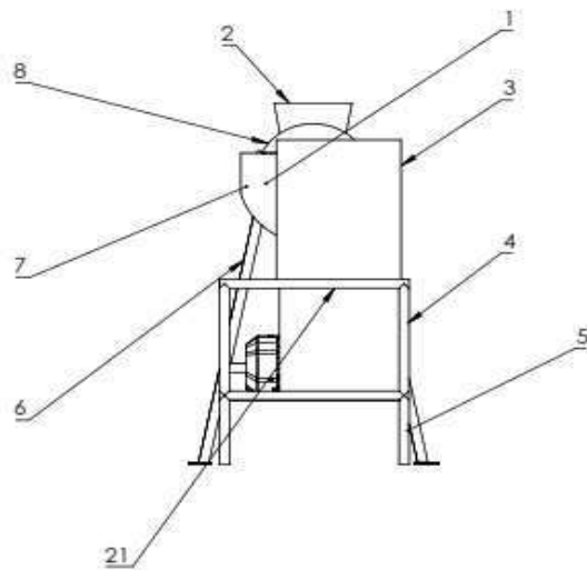
VISTA IZQUIERDA
