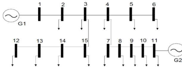
FIGURA 2. Sistema de distribución radial IEEE 15 nodos [21]
