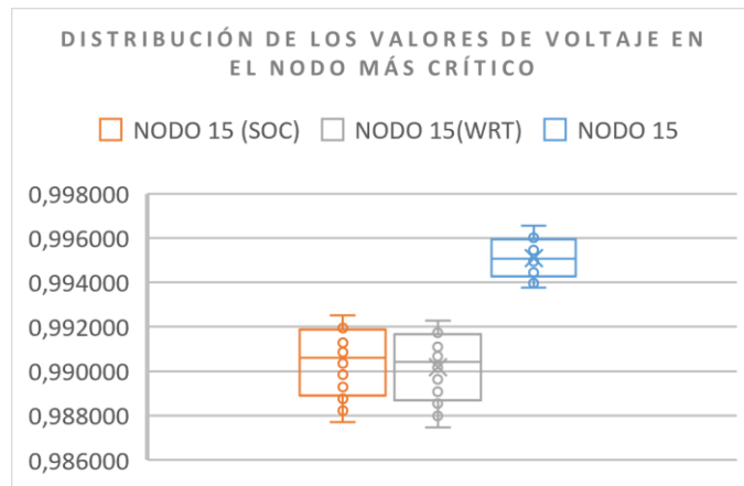
FIGURA 7. Distribución de voltajes del segundo orden cónico, Wirtinger y modelo no convexo en un periodo de 12 horas en el nodo más crítico.
