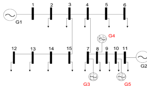
FIGURA 4. Sistema de distribución radial IEEE 15 nodos, incorporando nuevas unidades de generación.
