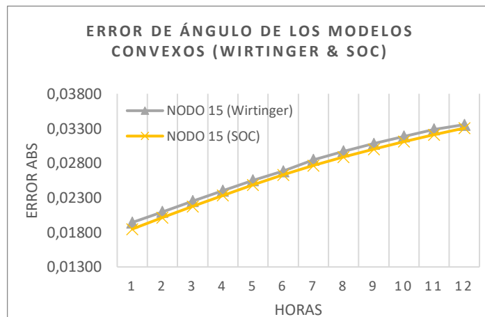
FIGURA 9. Error absoluto en ángulo de los modelos convexos frente al modelo no convexo en el nodo más crítico.
