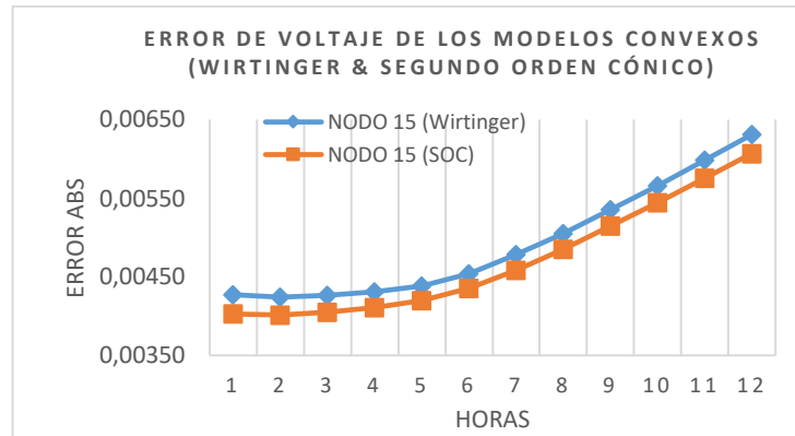
FIGURA 8. Error absoluto en voltaje de los modelos convexos frente al modelo no convexo en el nodo más crítico.
