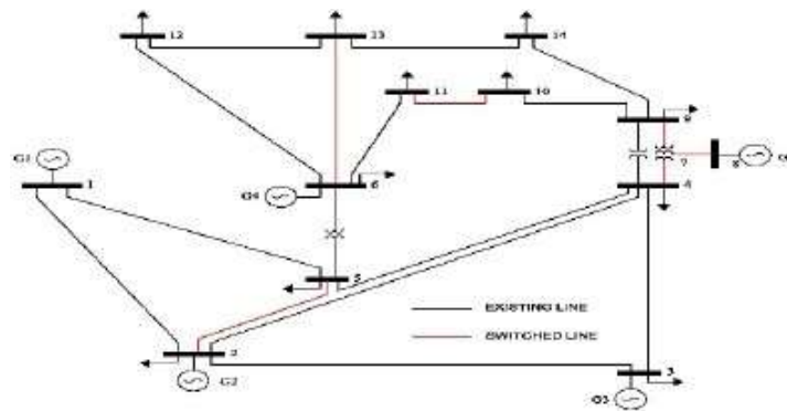
Figura 5: Sistema IEEE 14 Barras utilizando el criterio de conmutación de líneas de transmisión (OTS)
