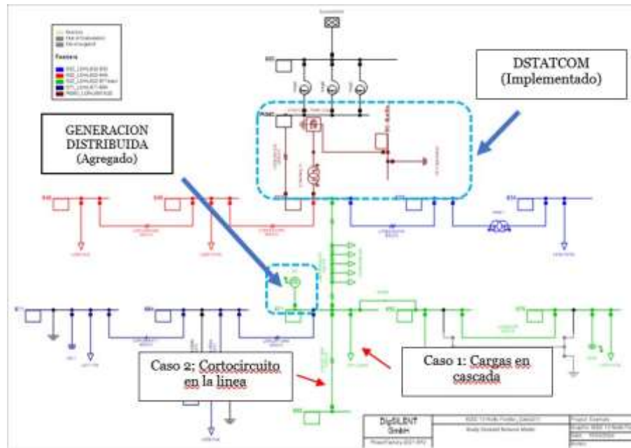
FIGURA 1. Diseño de DSTATCOM implementado en la red de 13 nodos de la IEEE
