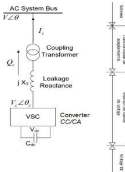
FIGURA 2. Modelo básico del STATCOM [15]
