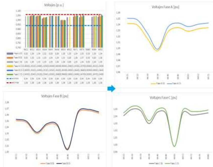
FIGURA 11. Grafica de la respuesta del perfil de voltaje SS y CS en nodos de 13 barras de la IEEE, fase A, B, C, caso 2
