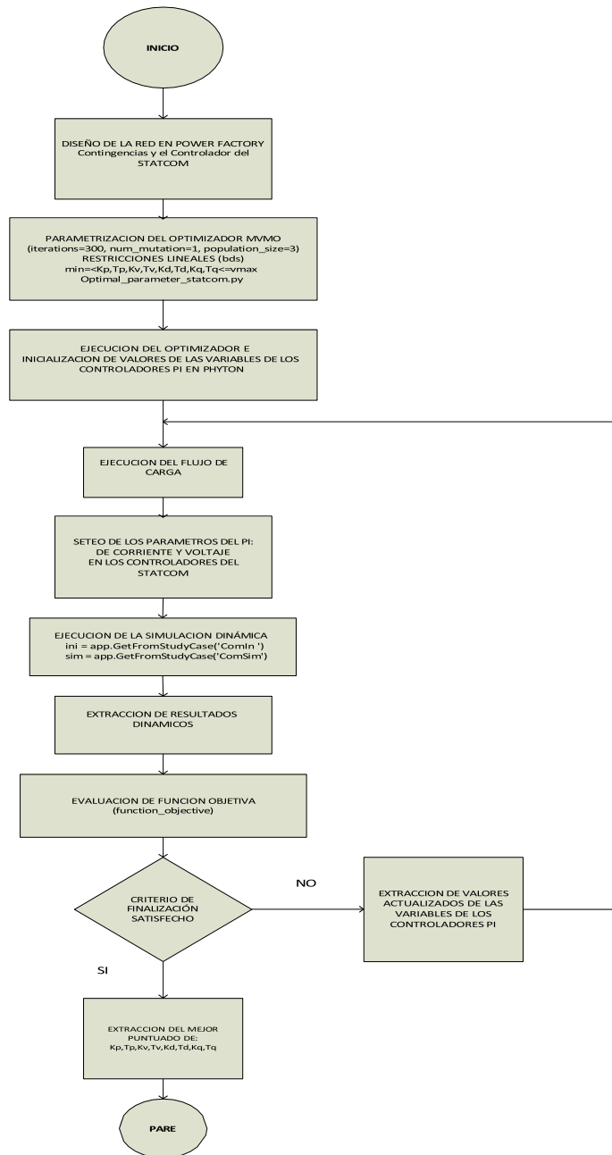
FIGURA 5. Metodología de sintonización dstatcom
