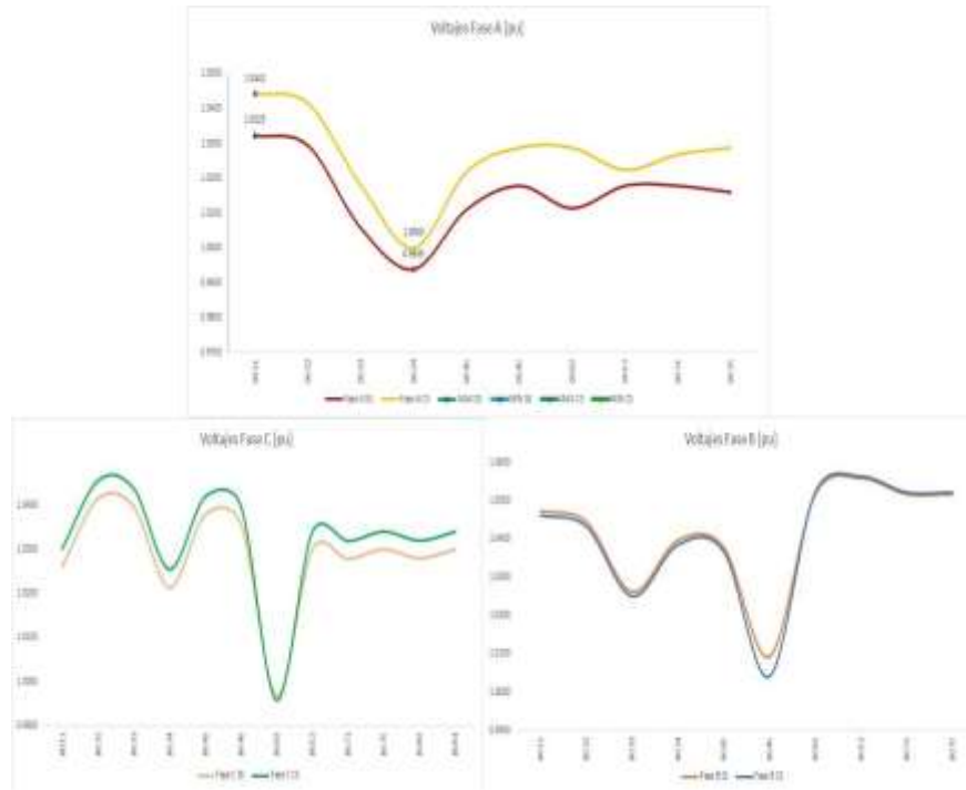
FIGURA 8. Grafica de la respuesta del perfil de voltaje SS y CS en nodos de 13 barras de la IEEE, fase A, B, C, caso 1
