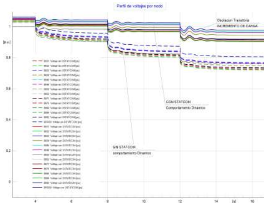
FIGURA 7. Comportamiento dinámico del voltaje de todos los nodos de la red de prueba, caso 1
