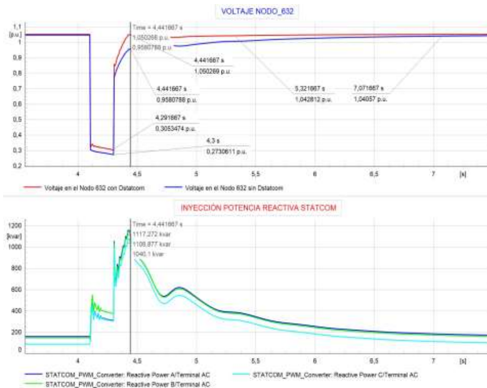
FIGURA 9. Comportamiento dinámico del voltaje e inyección de reactivos con evento de cortocircuito, con y sin dstatcom, nodo de incidencia 632
