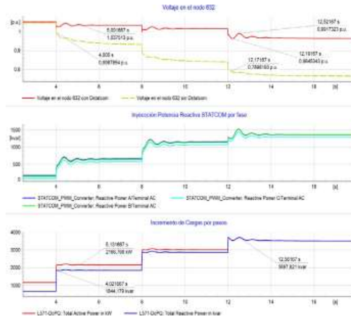
FIGURA 6. Comportamiento dinámico e inyección de reactivos con evento de incremento de carga en cascada, con y sin dstatcom, nodo de incidencia 632
