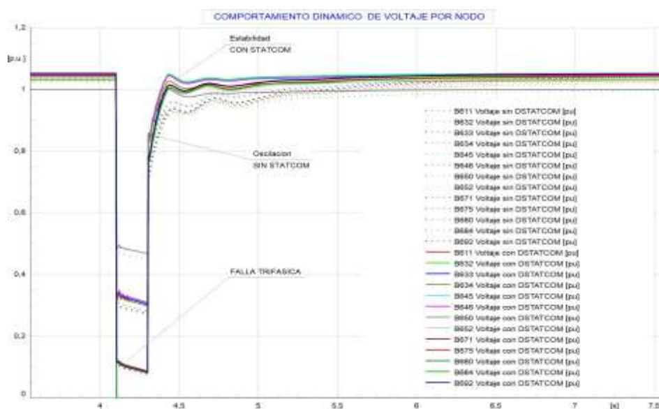
FIGURA 10. Comportamiento dinámico del voltaje de todos los nodos de la red de prueba, caso 2
