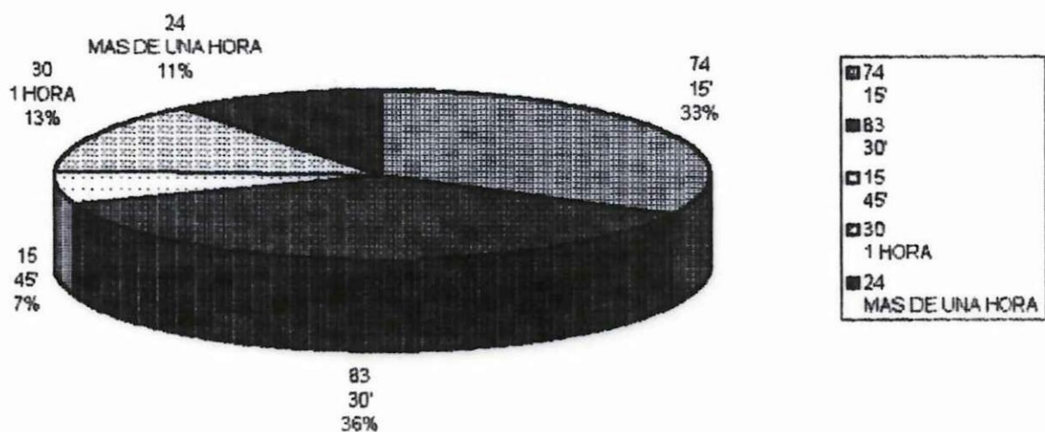
¿ CUANTO TIEMPO USTED DEDICA A LA LECTURA? GRAFICO # 5
